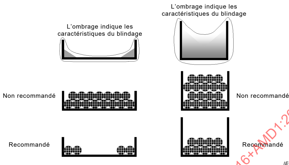
Figure H.4 – Dispositions des câbles dans des chemins de câbles métalliques
