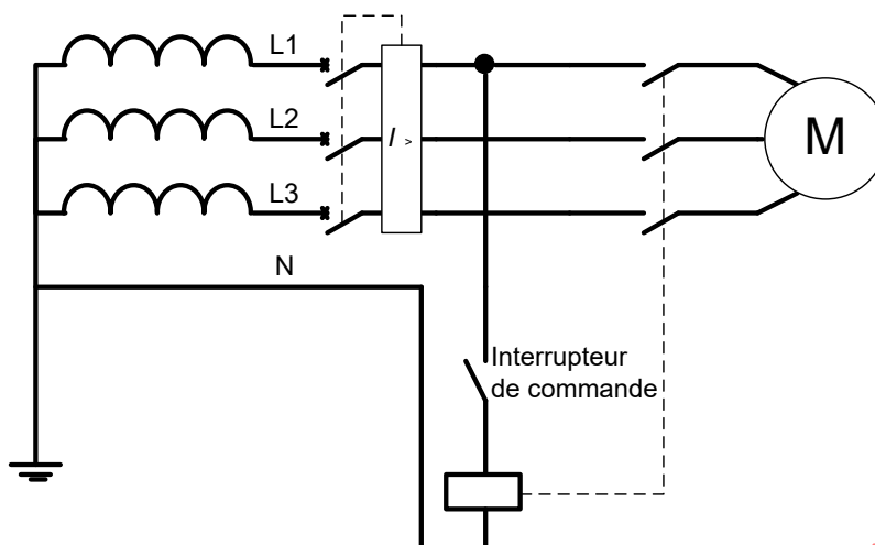
Figure 12 – Méthode d1a) Circuit de commande sans transformateur relié entre une phase et le neutre d'un réseau d'alimentation mis à la terre
