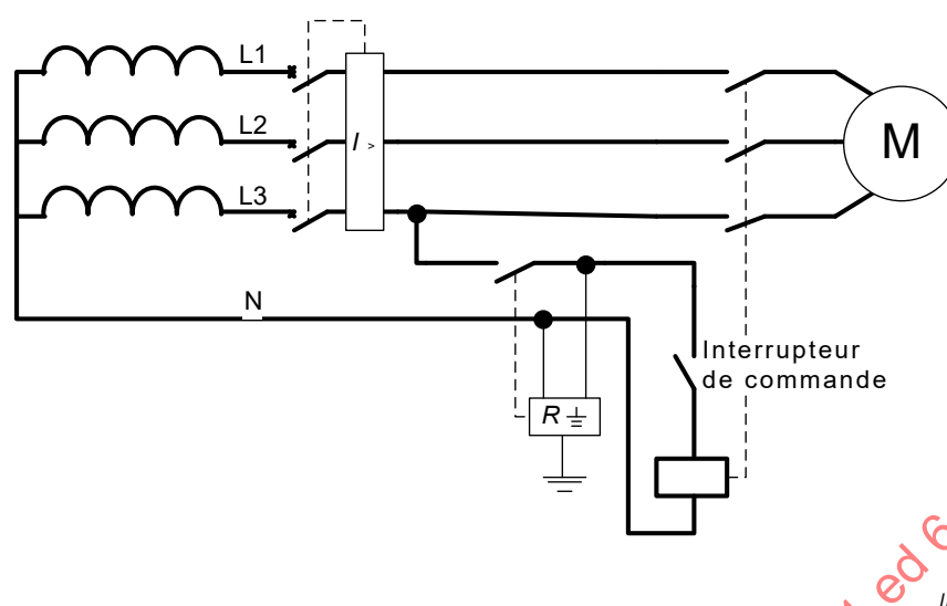
Figure 14 – Méthode d2a) Circuit de commande sans transformateur relié entre une phase et le neutre d'un réseau d'alimentation non mis à la terre
