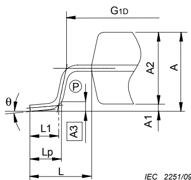
Figure 1d – Vue de côté du conducteur
