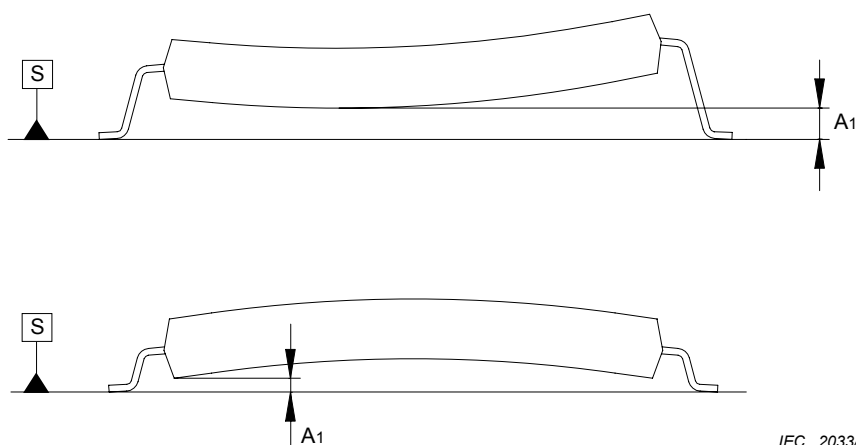
Figure 4 – Élévation
