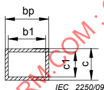
Figure 1c – Section de conducteur
