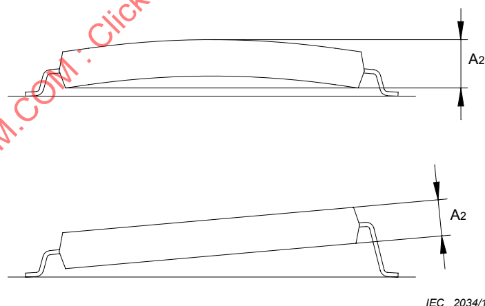
Figure 5 – Épaisseur du corps A2
