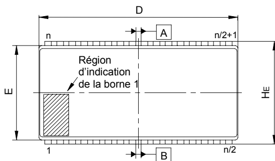
Figure A.9a - Vue de dessus
