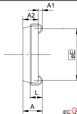
Figure A.9b - Vue de côté
