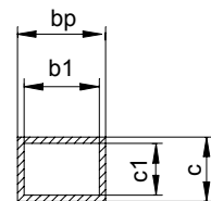
Figure A.9f - Section de conducteur
