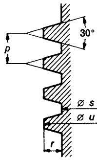
FIG. 3. — Détail du filetage. Detail of screw thread.
