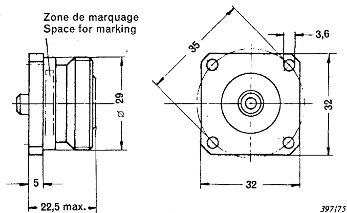
FIG. 8. — Embase (fixation au panneau par quatre trous avec cosse à souder) avec contact femelle. Fixed connector (4-hole panel mounting with solder bucket) with socket contact.
