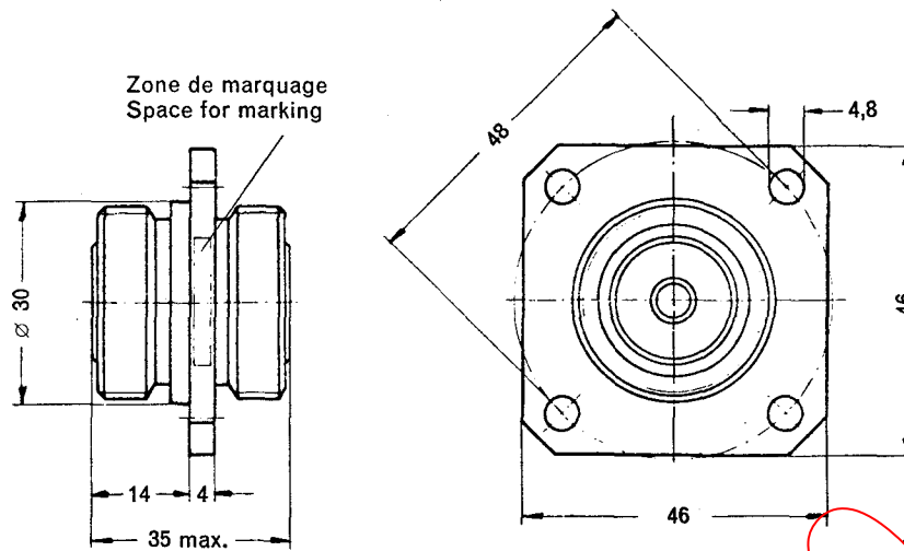
FIG. 12. — Raccord à platine (fixation au panneau par quatre trous) avec contacts femelle-femelle. Adaptor (4-hole panel mounting) with socket-socket contacts.
