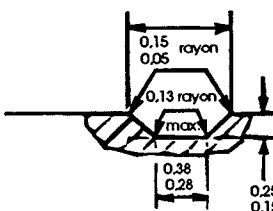
Figure 2d - Variante de la gorge d'accouplement
