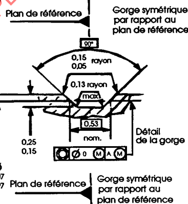
Figure 2c - Détails de la gorge d'accouplement
