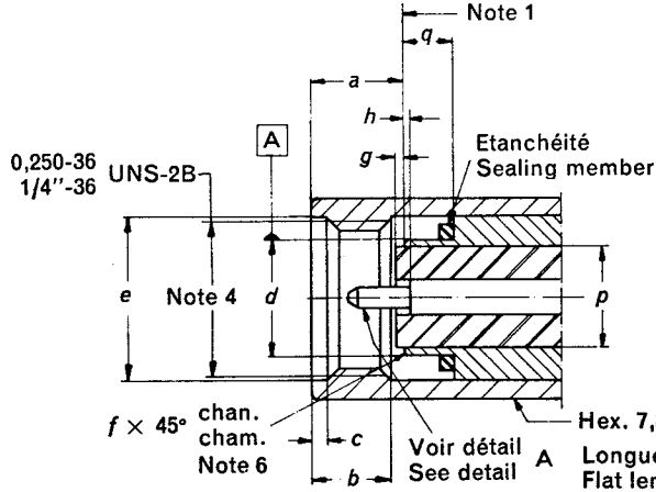
FIG. 1. — Connecteur avec contact central mâle (pour les dimensions, voir le tableau). Connector with pin centre contact (for dimensions, see table).
