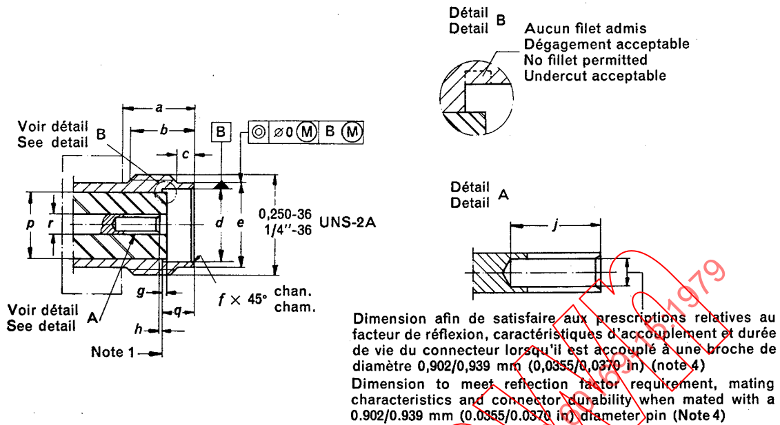
FIG. 2. — Connecteur avec contact central femelle (pour les dimensions, voir le tableau). Connector with socket centre contact (for dimensions, see table).
