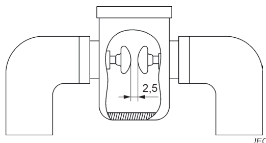
Figure 2 – Exemple de cellule d'essai avec des électrodes partiellement hémisphériques d'un rayon de 25 mm et d'un diamètre de 36 mm
