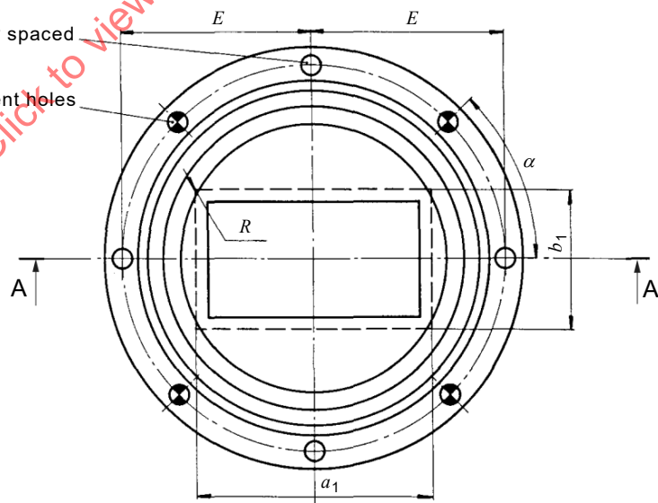
Figure 3 – Flange type A: 60154 IEC-AR 48
