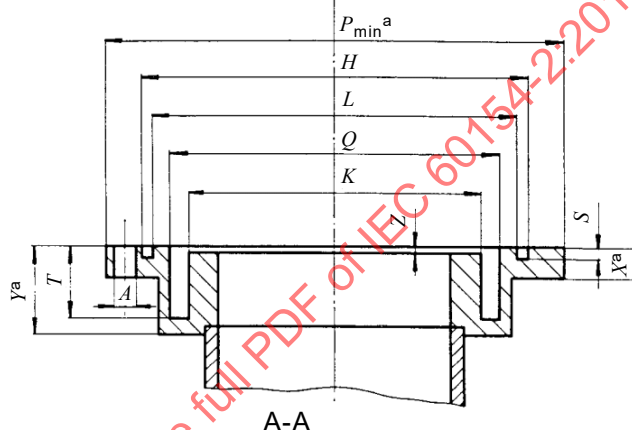
Bride modèle C 60154 IEC – CAR 32
