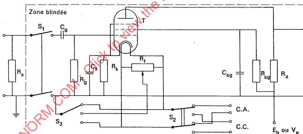
FIG. 2. — Circuit type pour mesurer le souffle et le ronflement
