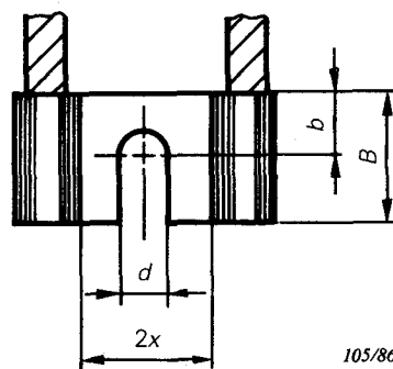
Cosse à deux bourrelets ouverte
