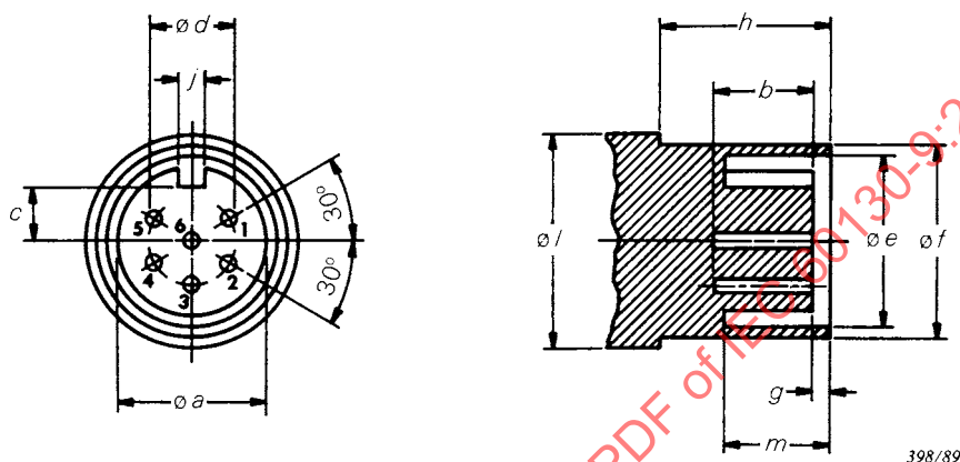
Figure 19 – Fiche 60130-9 IEC-18
