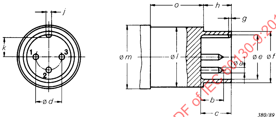
Figure 1 – Fiche 60130-9 IEC-01
