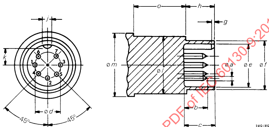
Figure 10 – Fiche 60130-9 IEC-10
