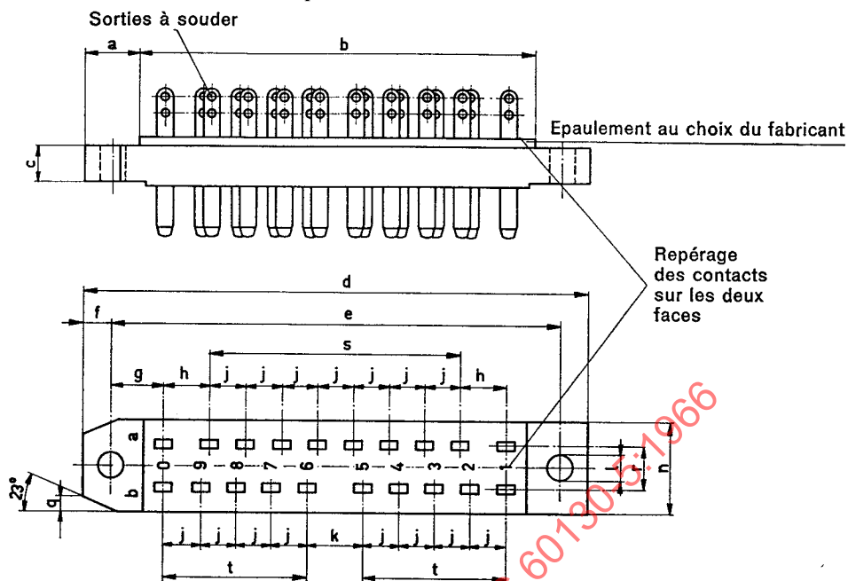
FIG. 1a). — Connecteur mâle.
