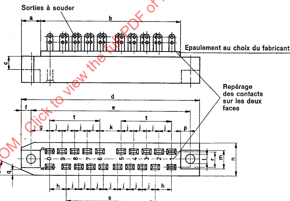
FIG. 1b). — Connecteur femelle.
