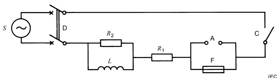
Figure 6 – Circuit d'essai caractéristique utilisé pour les essais du pouvoir de coupure des éléments de remplacement à haut pouvoir de coupure (voir 9.3)
