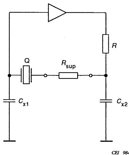
Figure A.2 – Réseau d'oscillateur avec R et R_{\text{sup}}
