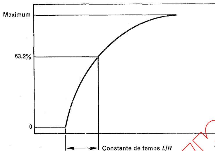
FIG. 2. — Oscillogramme
