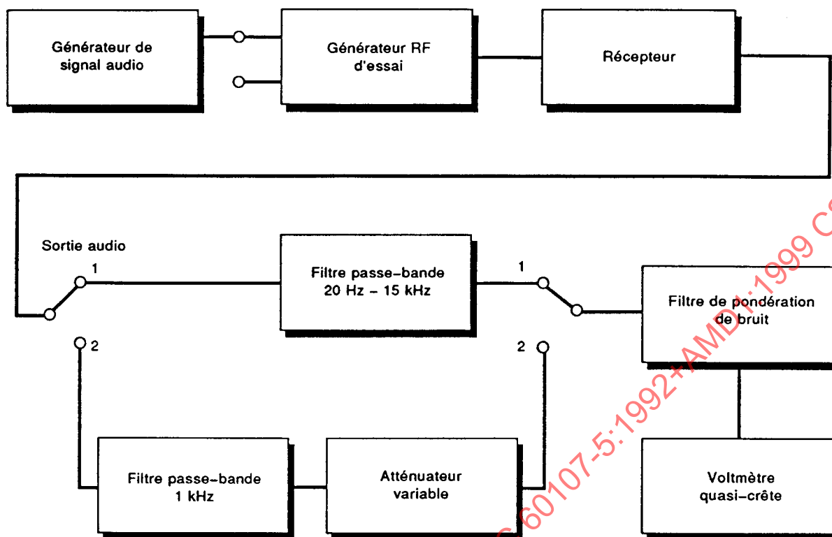
Figure 5 – Disposition pour les mesures du rapport signal sur bruit
