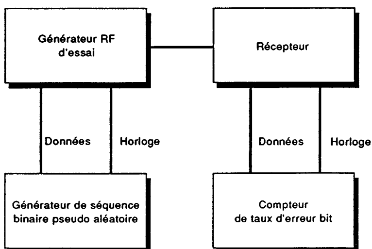
Figure 3 – Disposition pour les mesures du taux d'erreur bit
