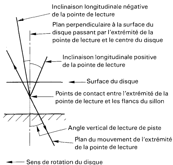
FIG. 1a. – Sillon vu de la pointe de lecture en direction du centre du disque (voir paragraphe 8.1).
