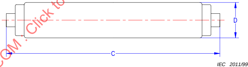
Culot R17d (voir feuille 7004-56 de la CEI 60061-1)
