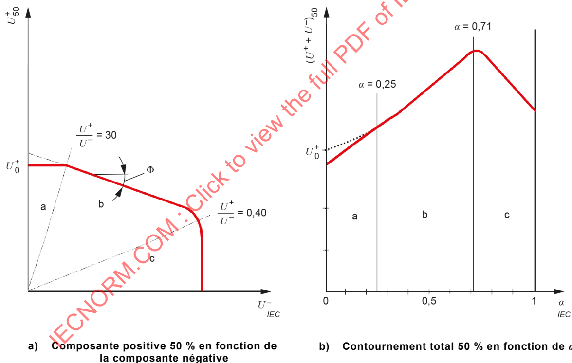
Figure C.4 – Configuration schématique de l'isolation entre phases et phase-terre
