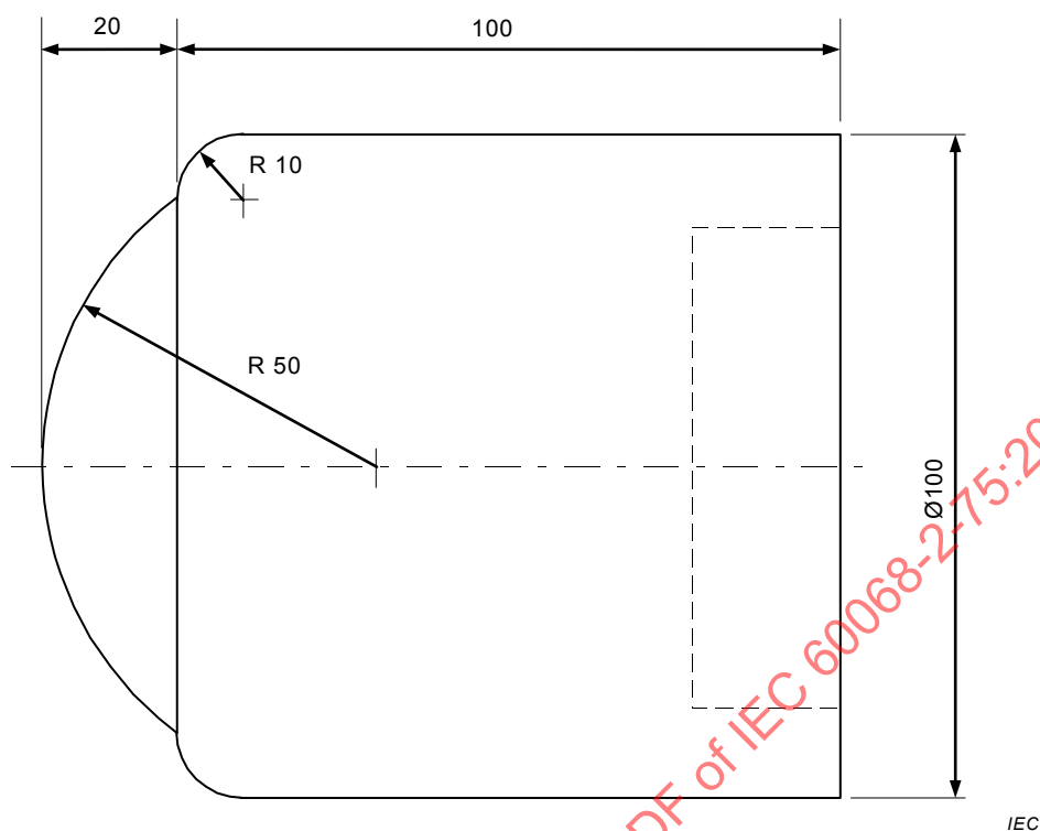
Figure A.5 – Exemple de pièce de frappe pour une valeur 20 J
