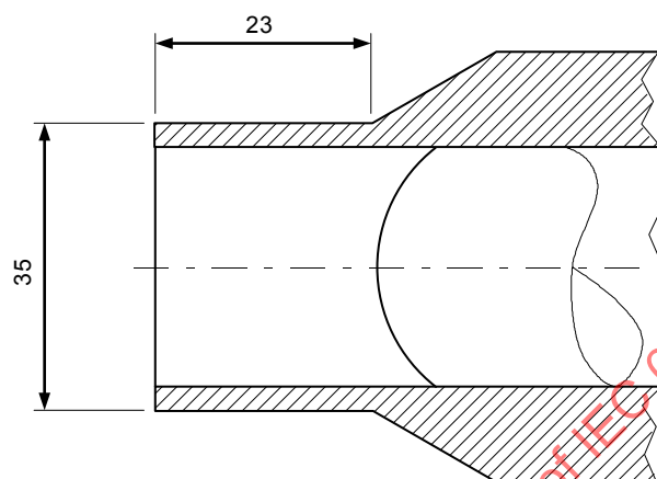
Figure 3 – Forme de la tête de déclenchement pour 2 J
