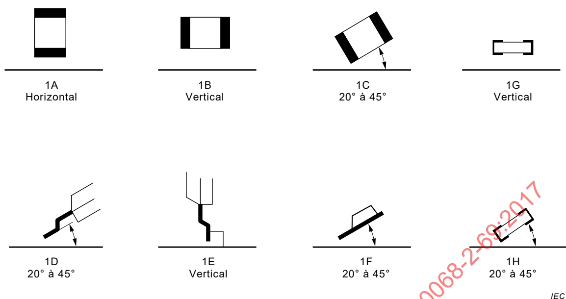
a) – Exemples d'immersion A à H
