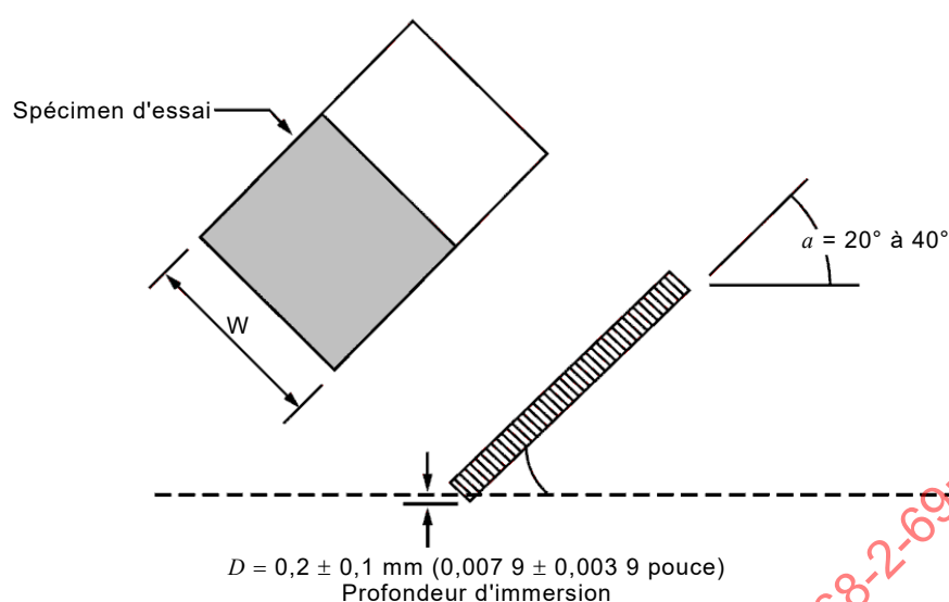
Figure 6 – Immersion de cartes imprimées
