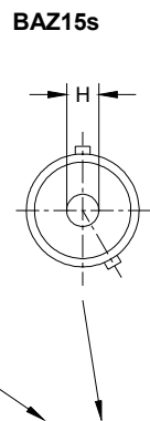
All other dimensions as for BAZ15d Toutes les autres dimensions sont les mêmes que pour BAZ15d
