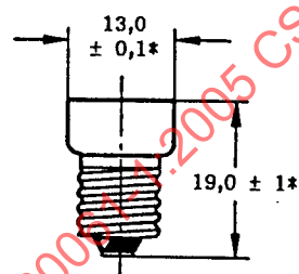
E10/19x13
