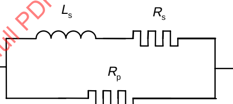
Figure A.1 – Schéma de la charge inductive pour les essais de performance en régime transitoire
