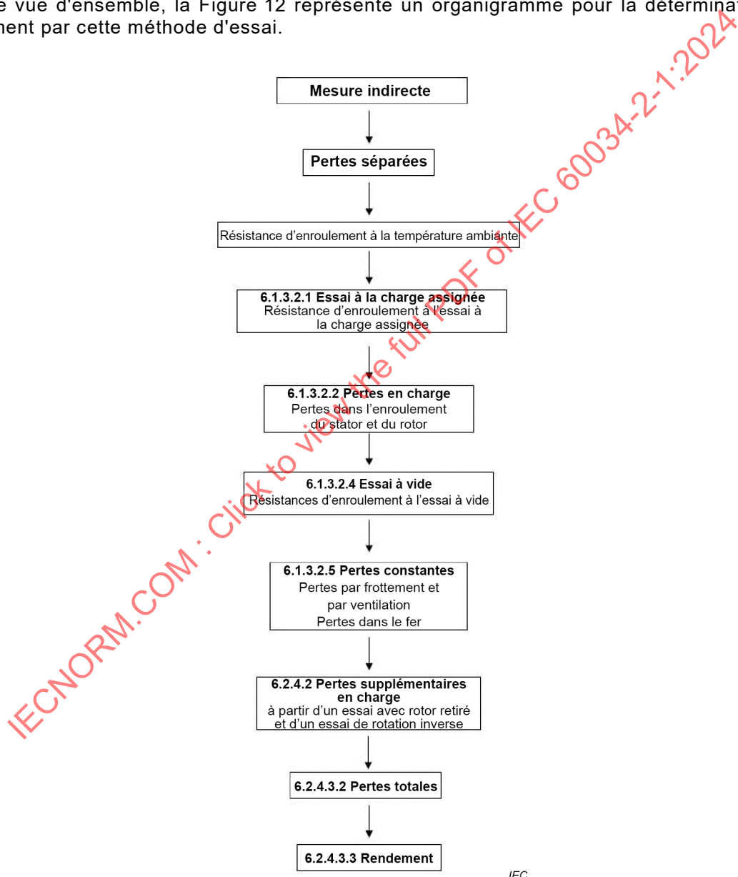
Figure 12 – Détermination du rendement selon la méthode 2-1-1F
