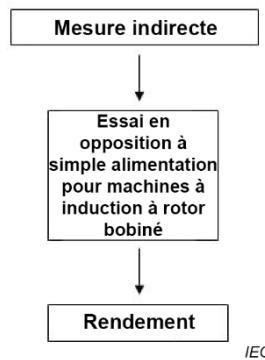
Figure 11 – Détermination du rendement selon la méthode 2-1-1E
