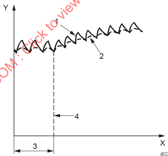
Figure 1 – Exemple de surcharge thermique à évolution lente et de protection thermique directe
