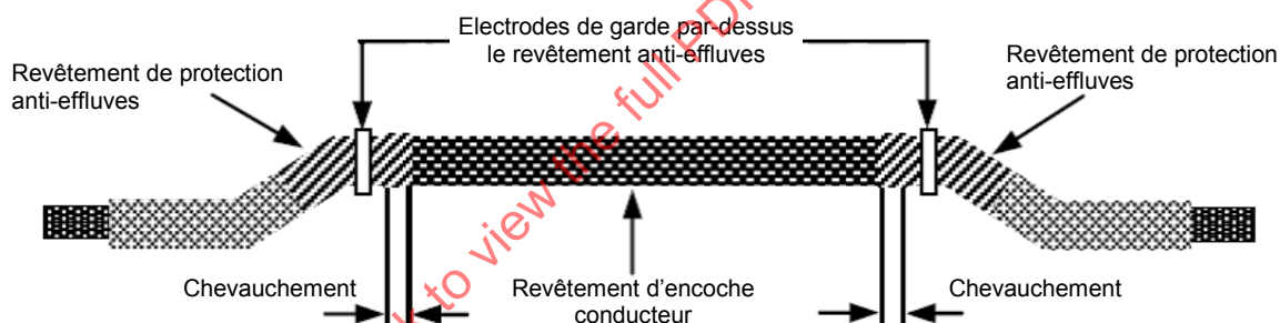
Figure 9 – Application d'électrodes à anneau de garde sur un revêtement de protection anti-effluves
