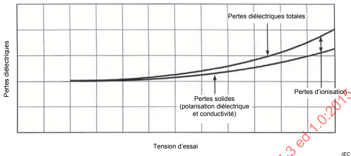
Figure 3 – Pertes diélectriques avec tension croissante (schéma)
