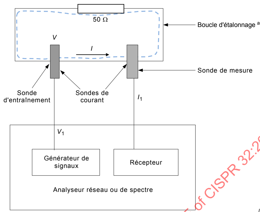
Figure C.6 – Montage d'étalonnage
