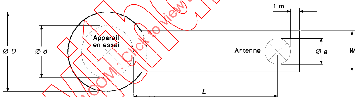
Figure 2 – Caractéristiques minimales d'un autre emplacement d'essai
