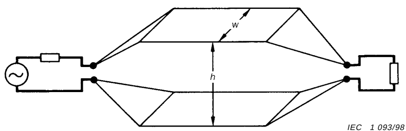
Figure 1 – Dispositif TEM à ligne ouverte: configuration de base (voir 5.2.2)
