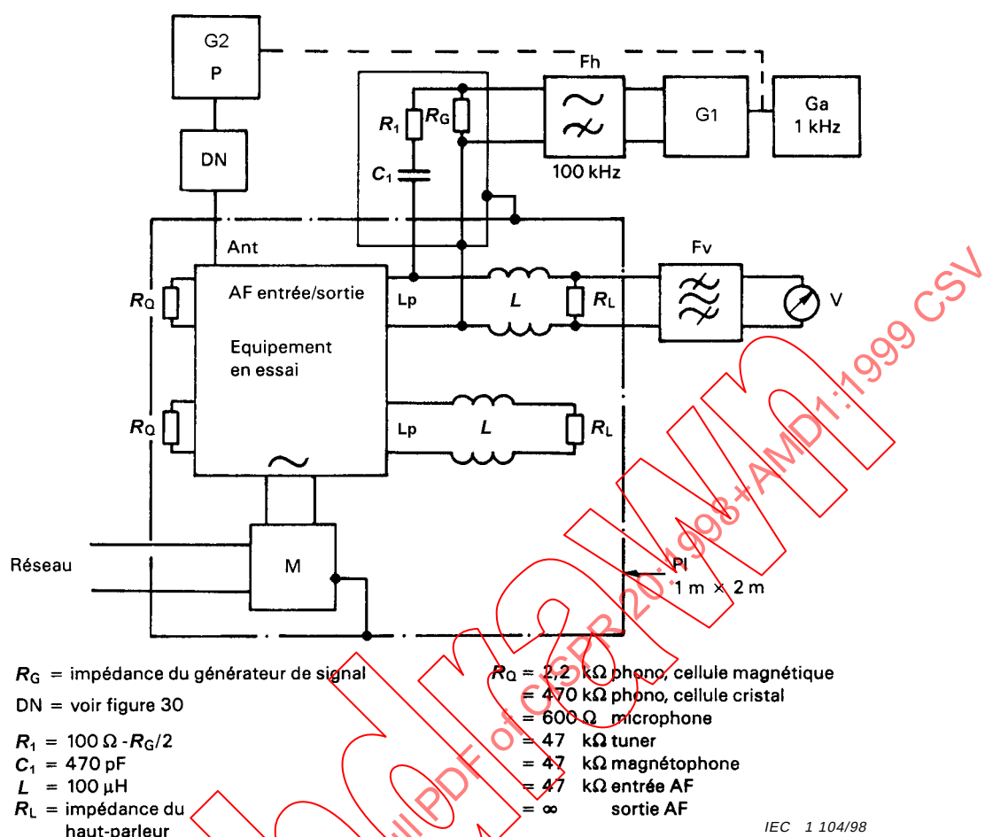
Figure 22 – Dispositif de mesure de l'essai d'immunité par la méthode d'injection de tension (bornes du haut-parleur) (voir 5.5.2)
