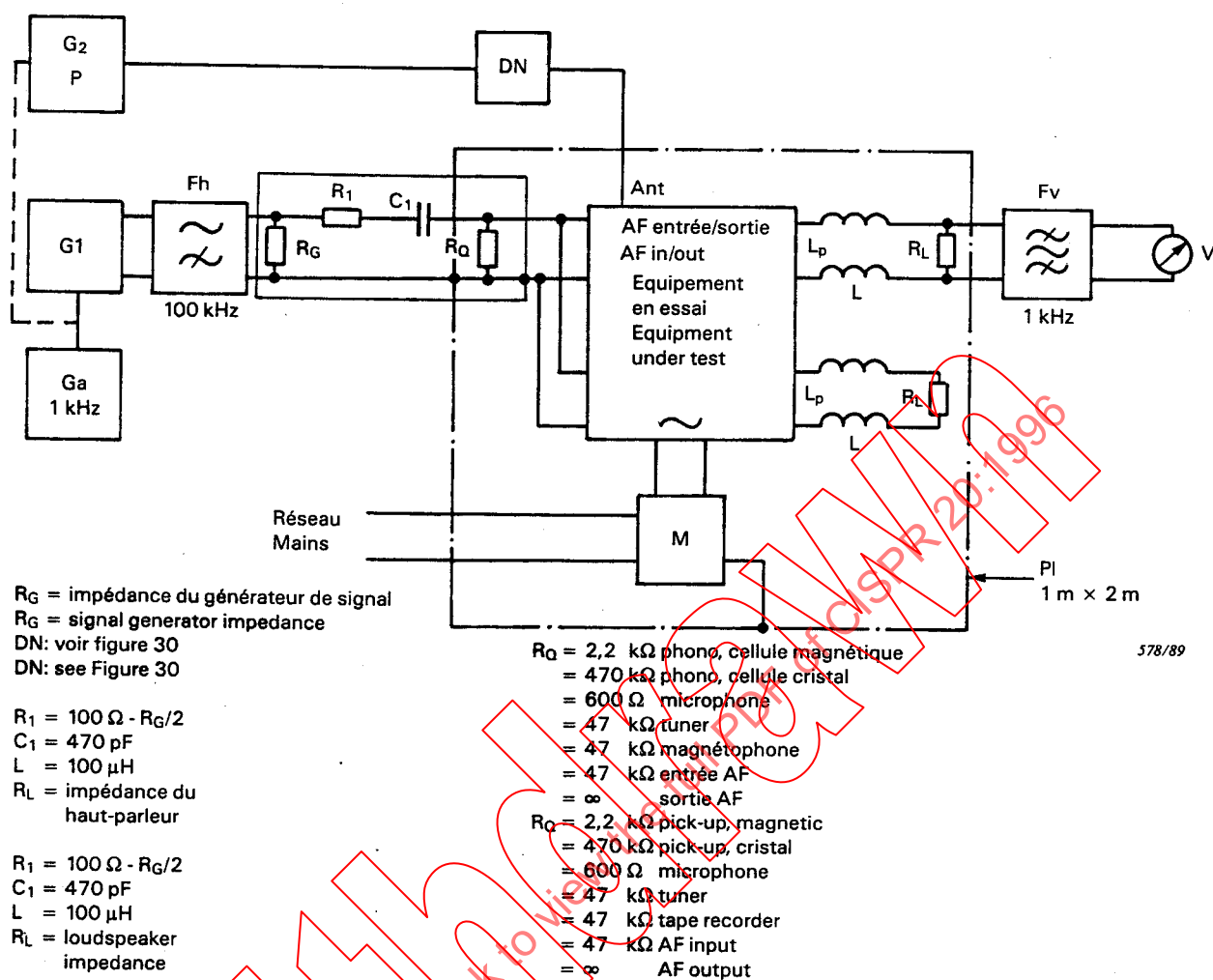
Figure 21 – Dispositif de mesure de l'essai d'immunité par la méthode d'injection de tension (bornes d'entrée/sortie audio (voir 5.5.2)) Measurement set-up for the immunity test by the voltage-injection method (input/output audio terminals) (see 5.5.2)
