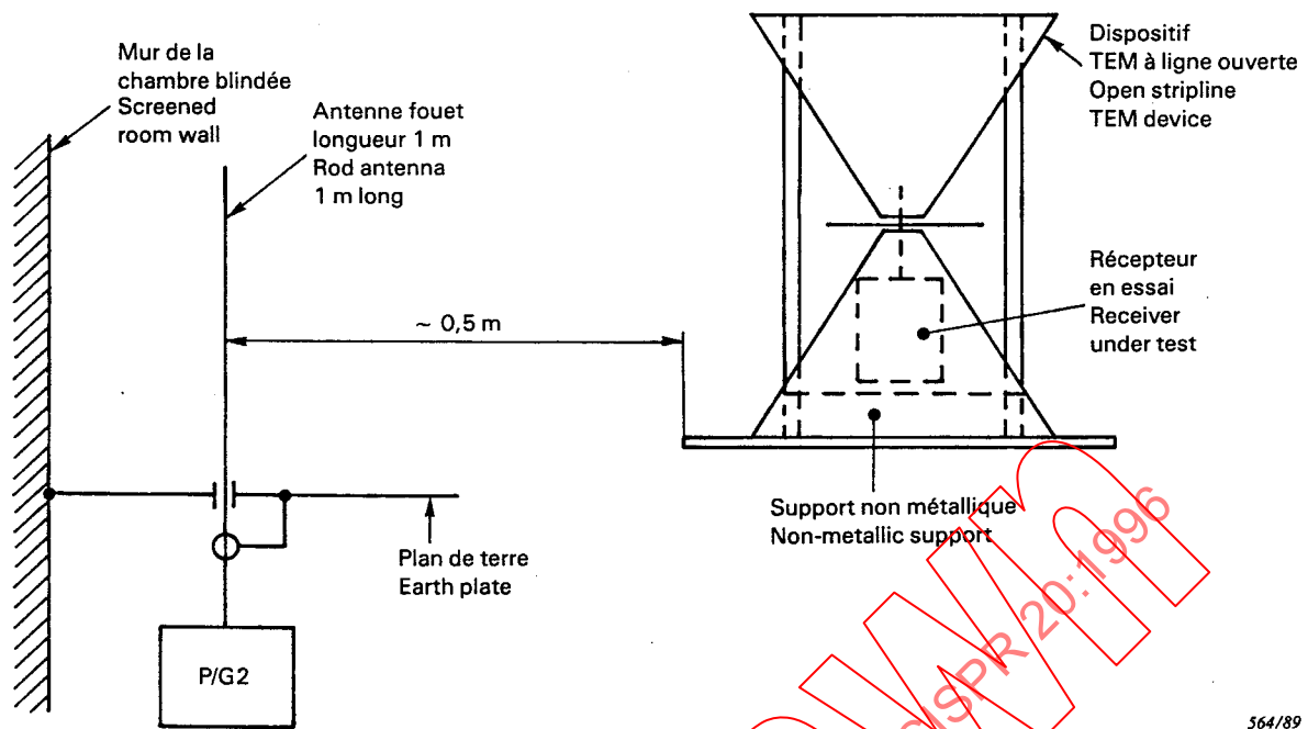
Figure 7 – Dispositif de mesure pour l'immunité de récepteurs de radiodiffusion non équipée de borne antenne (autre dispositif pour la figure 6 quand un dispositif TEM à ligne ouverte est utilisé) voir 5.2.3.2)
