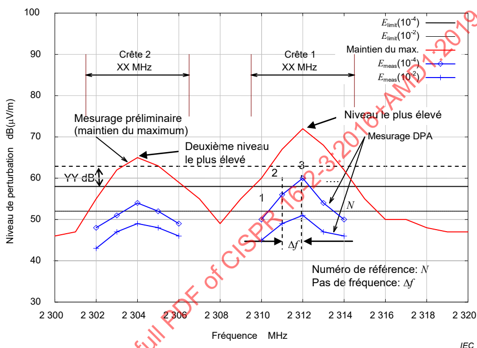
Figure D.1 – Exemple de mesurage de DPA par la Méthode 1 pour des perturbations fluctuantes
