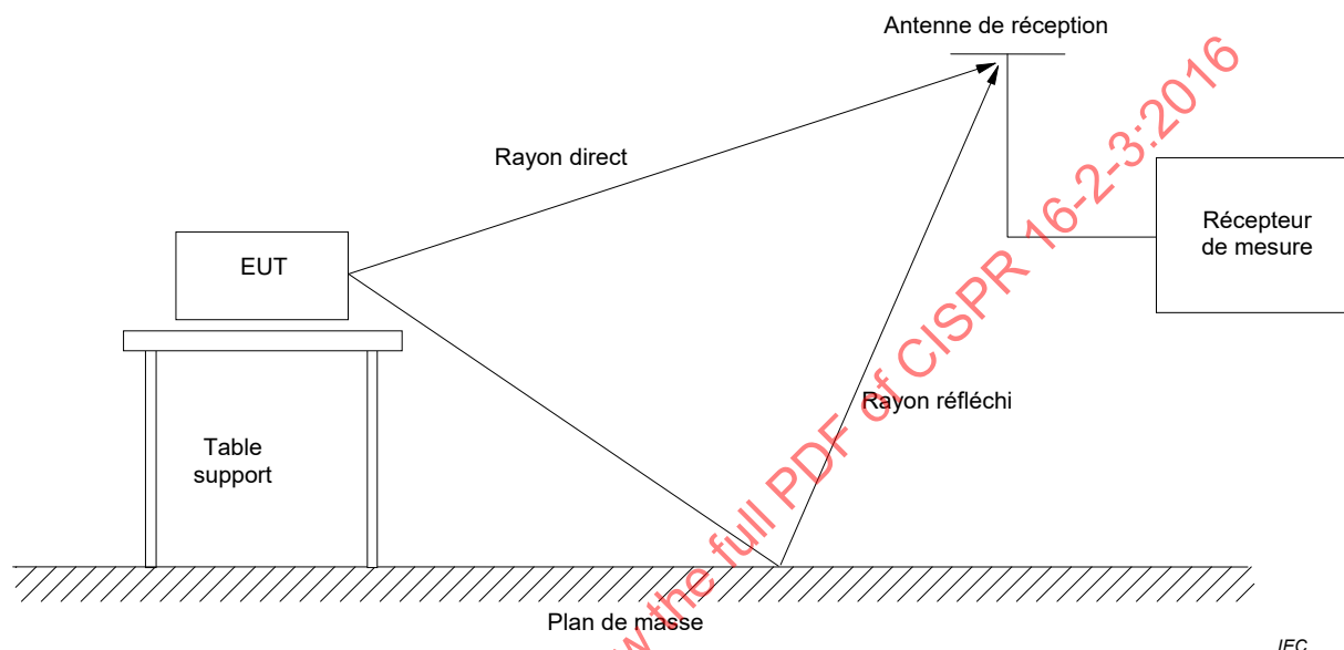
Figure 10 – Concept des mesurages de l'amplitude de champ électrique effectués sur un emplacement d'essai en espace libre (OATS) ou dans une chambre semi-anéchoïque (SAC) représentant les rayons directs et réfléchis arrivant sur l'antenne de réception
