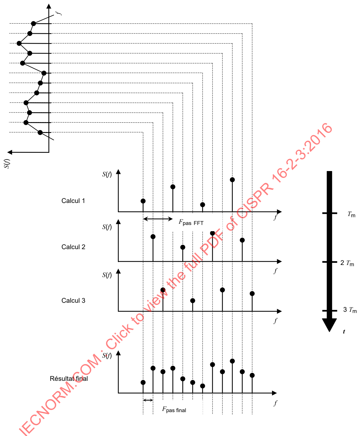
Figure 6 – Résolution en fréquence améliorée au moyen d'un appareil de mesure à FFT
