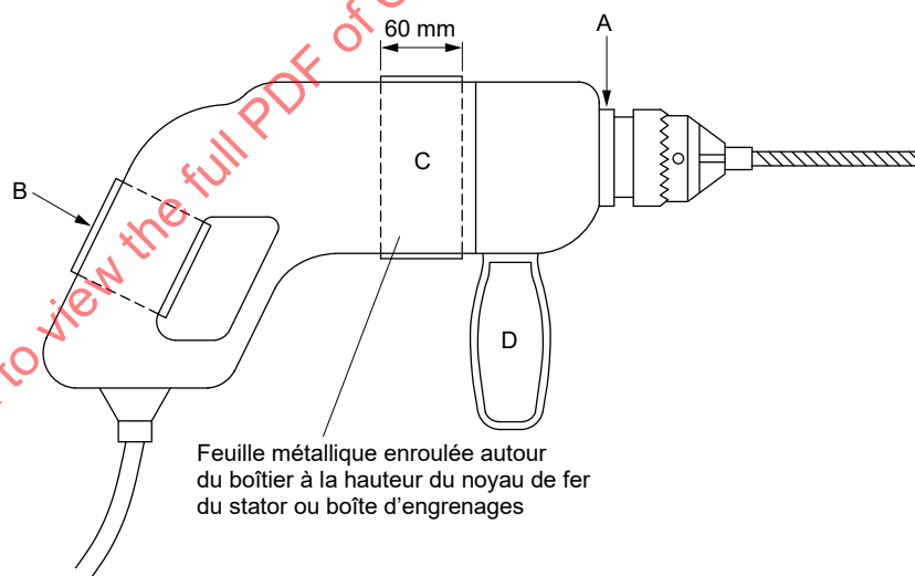
Figure 18 – Perceuse électrique portative avec main artificielle
