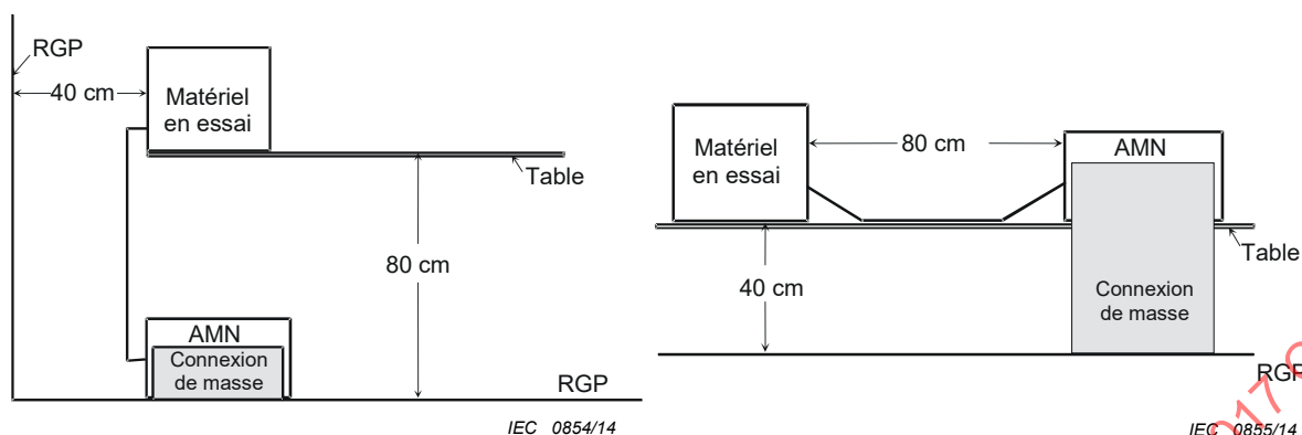
a) b) Figure 10 – Montage de matériel en essai et de réseau AMN à 40 cm avec a) RGP vertical et b) RGP horizontal
