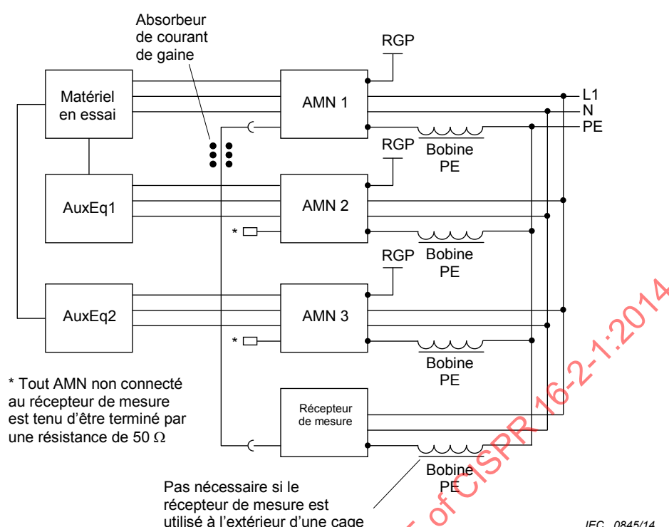
Figure 1 – Exemple d'un montage d'essai recommandé avec bobines PE, trois réseaux fictifs d'alimentation et un absorbeur de courant de gaine sur le câble RF
