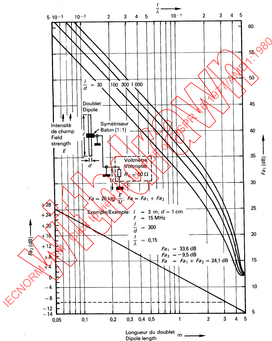
FIG. 42. — Facteurs d'antenne des doublets courts pour R_L = 50 \Omega . Short dipole aerial factors for R_L = 50 \Omega .
