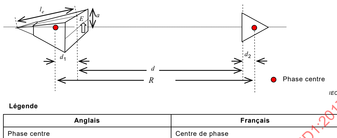
Figure 15 – Distance de séparation par rapport au centre de phase des antennes cornes (voir détails en [49])
