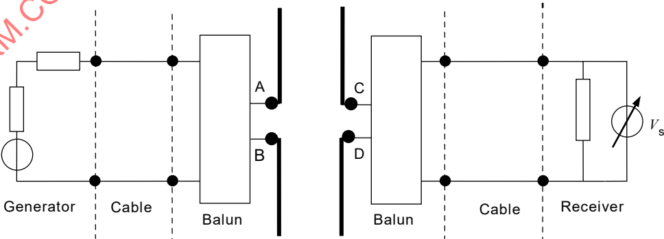
Figure 3 – Détermination de V_{r1}(f) ou V_{r2}(f)
