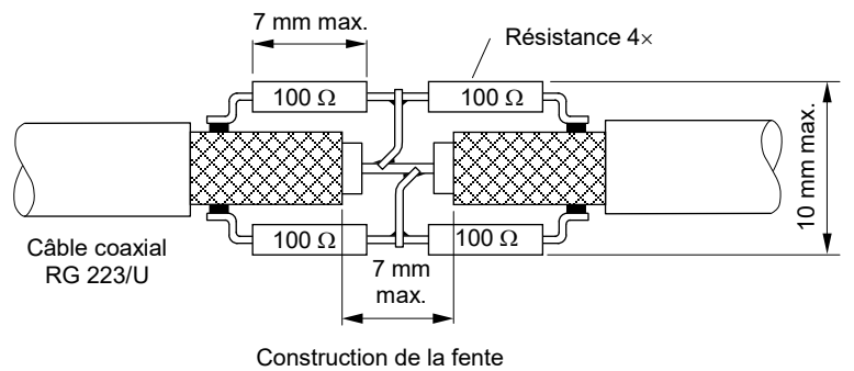
Figure C.3 – Construction de la fente de l'antenne
