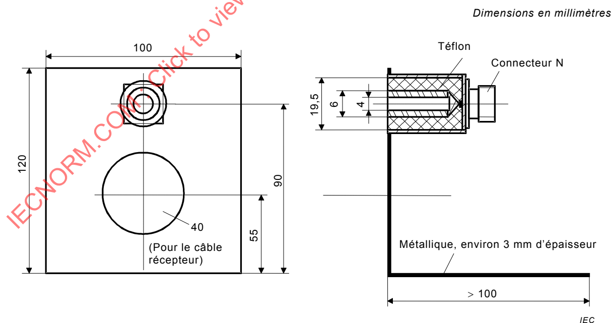
Figure B.5a – Flasque verticale de type A (côté SAD)
