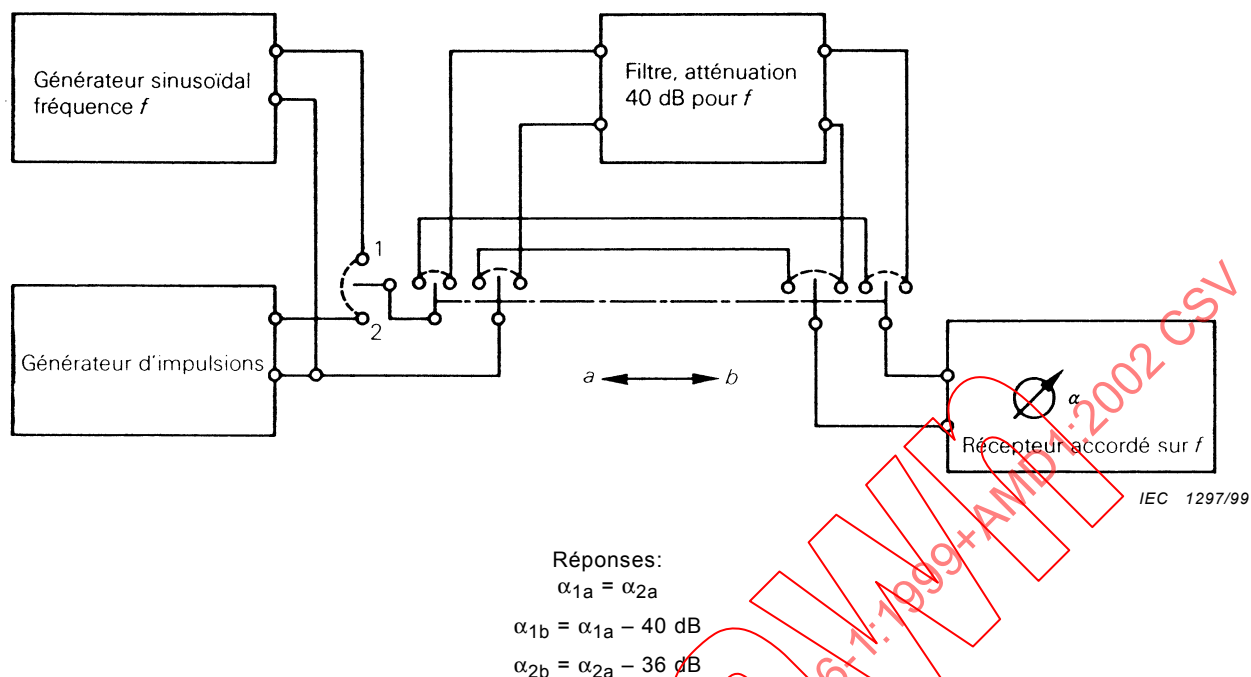
Figure 3 – Schéma pour l'essai des effets d'intermodulation (voir 4.1.6)
