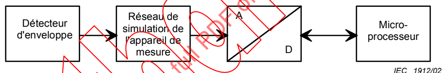
Figure 60 – Schéma d'un détecteur de valeur moyenne
