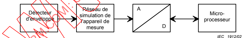
Figure 5 – Schéma fonctionnel d'un détecteur de valeur moyenne
