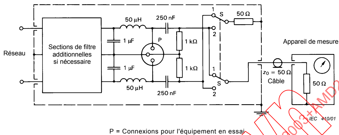
Figure 3 – Exemple d'un réseau fictif d'alimentation 50 Ω-50 μH (voir 5.3.1)
