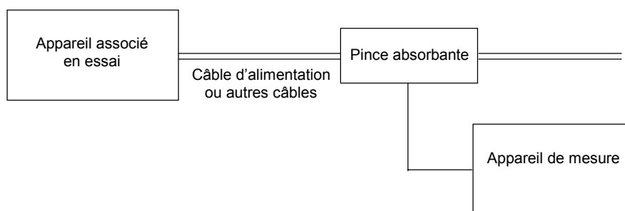
Figure 10 – Disposition de mesure de la puissance perturbatrice des équipements associés (à l'exclusion des magnétoscopes) (voir 5.6.3)
