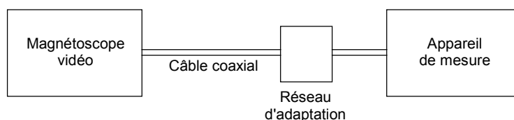
Figure 9 – Disposition de mesure du signal utile et de la tension perturbatrice aux bornes de la sortie RF des magnétoscopes vidéo (voir 5.5.2)
