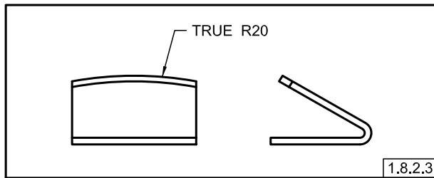
Fig. 1-26 True Radius
