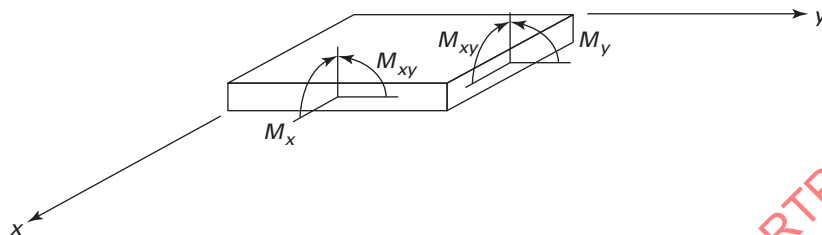
Fig. M3-1 Moment Resultants
