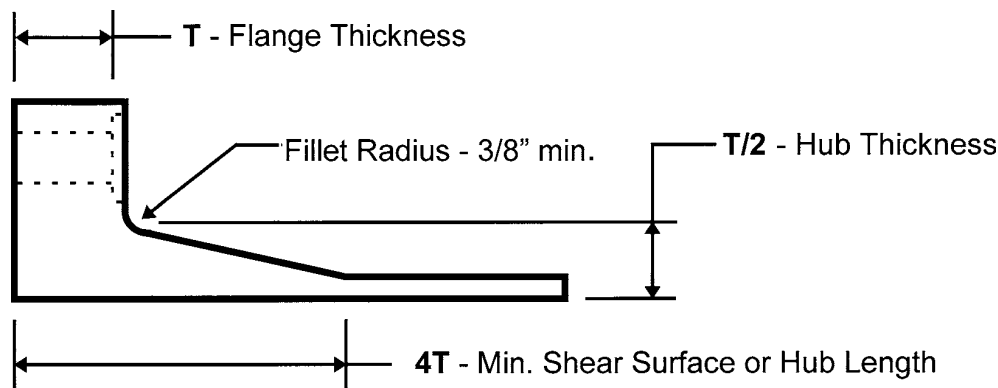
FIG. 1 Flange Dimensions
