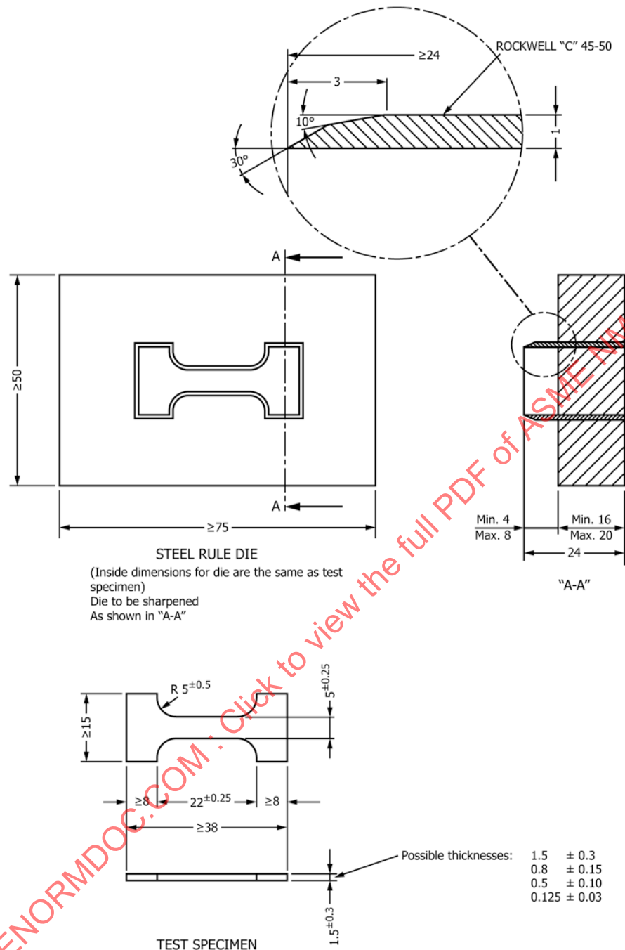
FIG. 11 Microtensile Die
