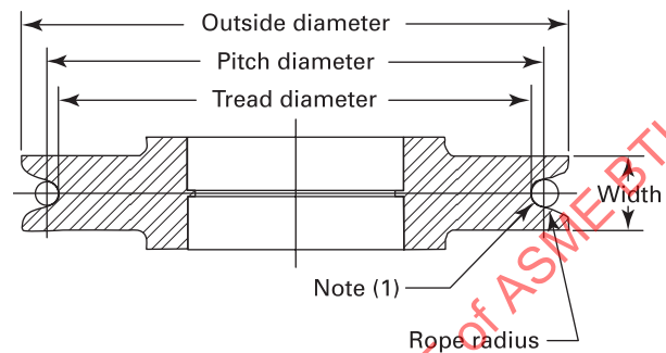
Fig. 4-2.6-1 Sheave Dimensions
